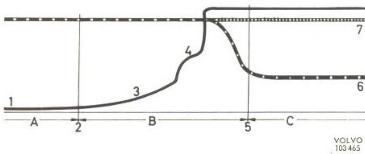
Bild 13. Tryck och varvtal vid inkoppling av överväxel
