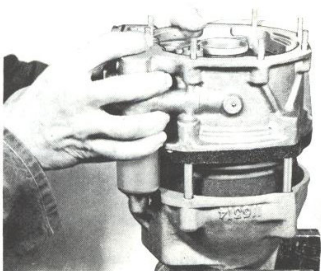
Bild 22. Isärtagning av överväxel
