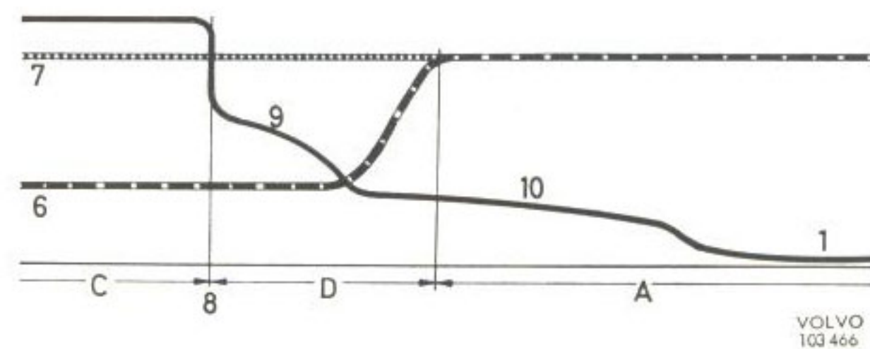
Bild 14. Tryck och varvtal vid urkoppling av överväxel
