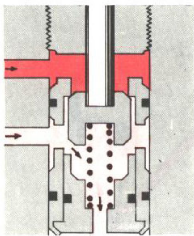
Bild 8. Manöverventil vid direktväxel
