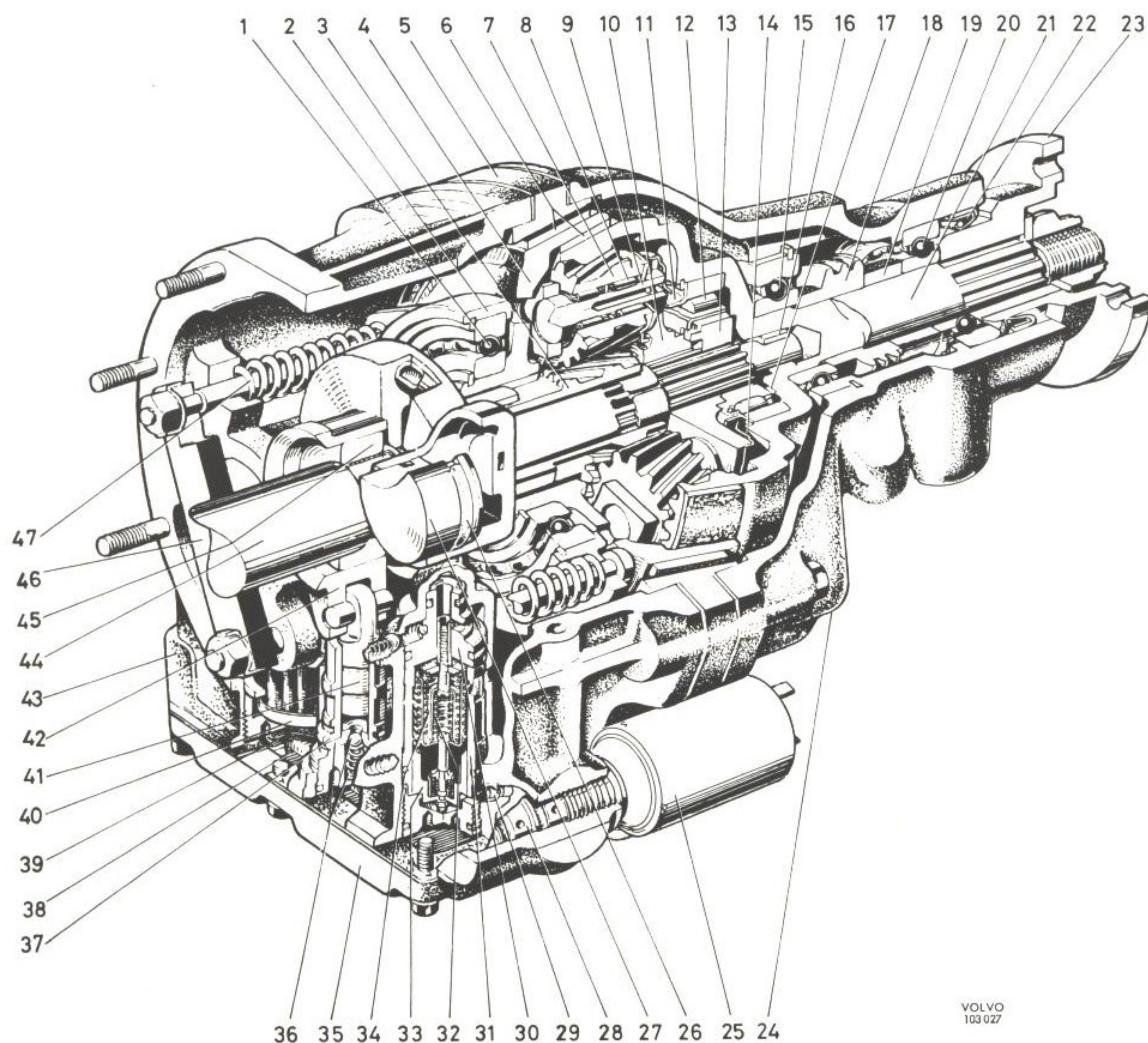
Bild 16. Överväxel
