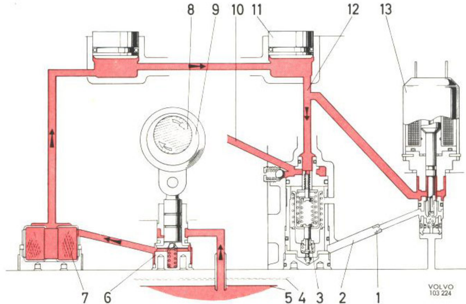
Bild 7. Funktion vid direktväxel
