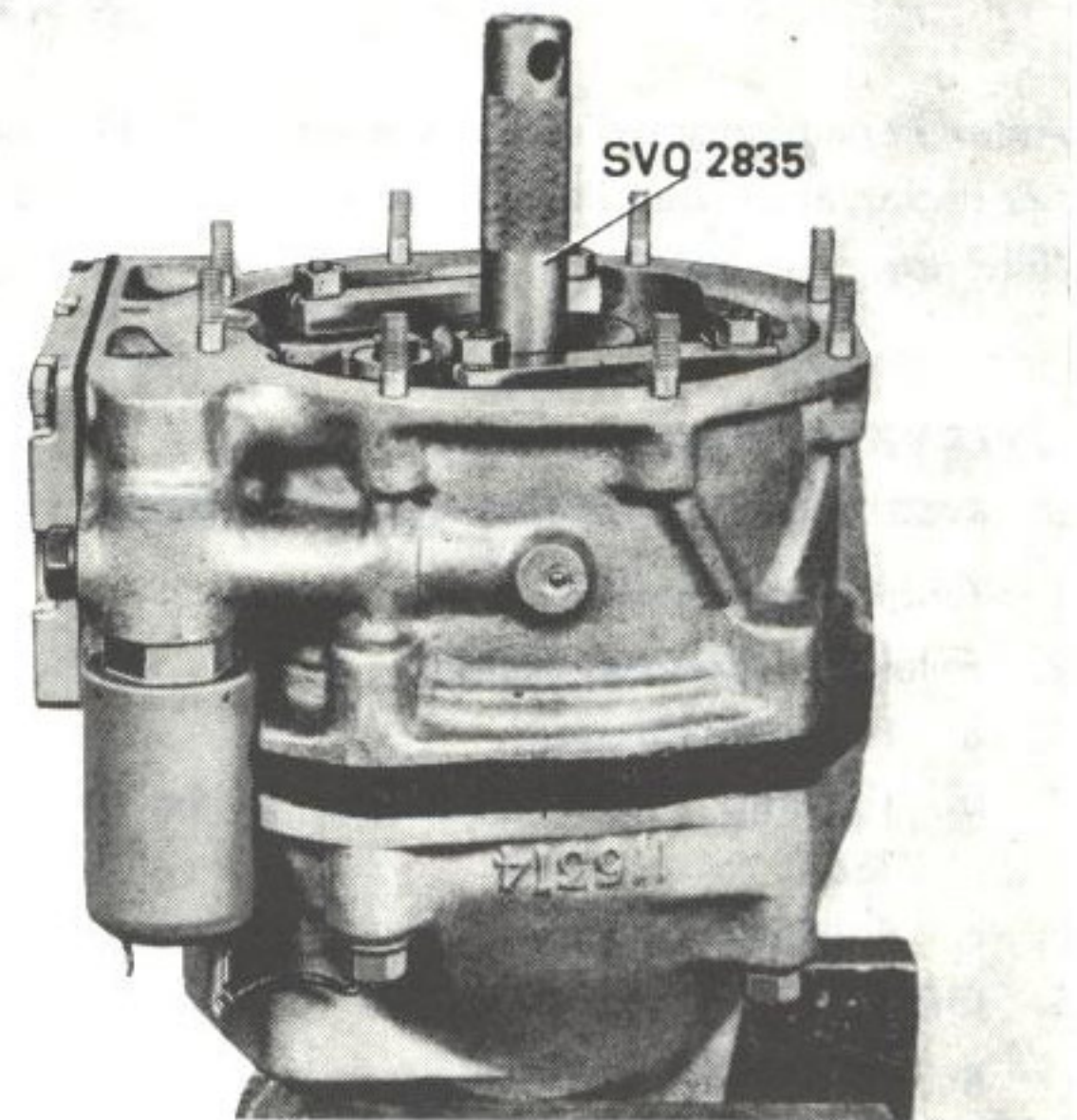
Bild 34. Montering av främre hushalva
