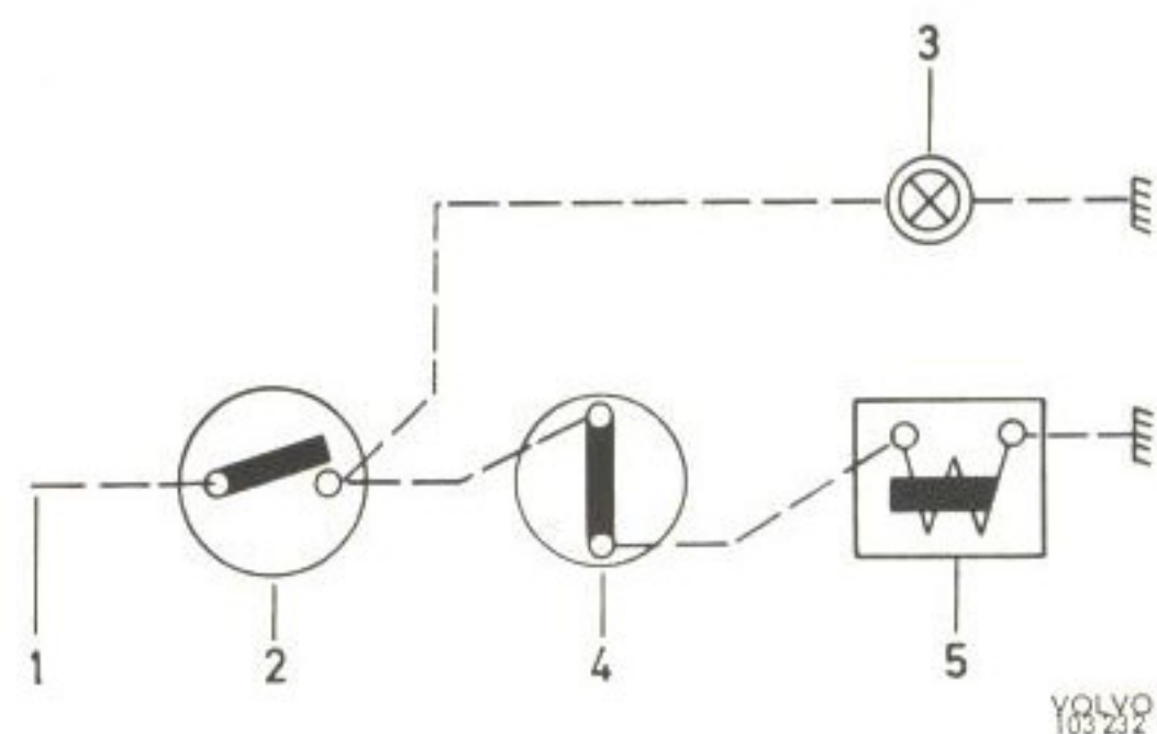
Bild 4. Elektriskt kopplingschema
