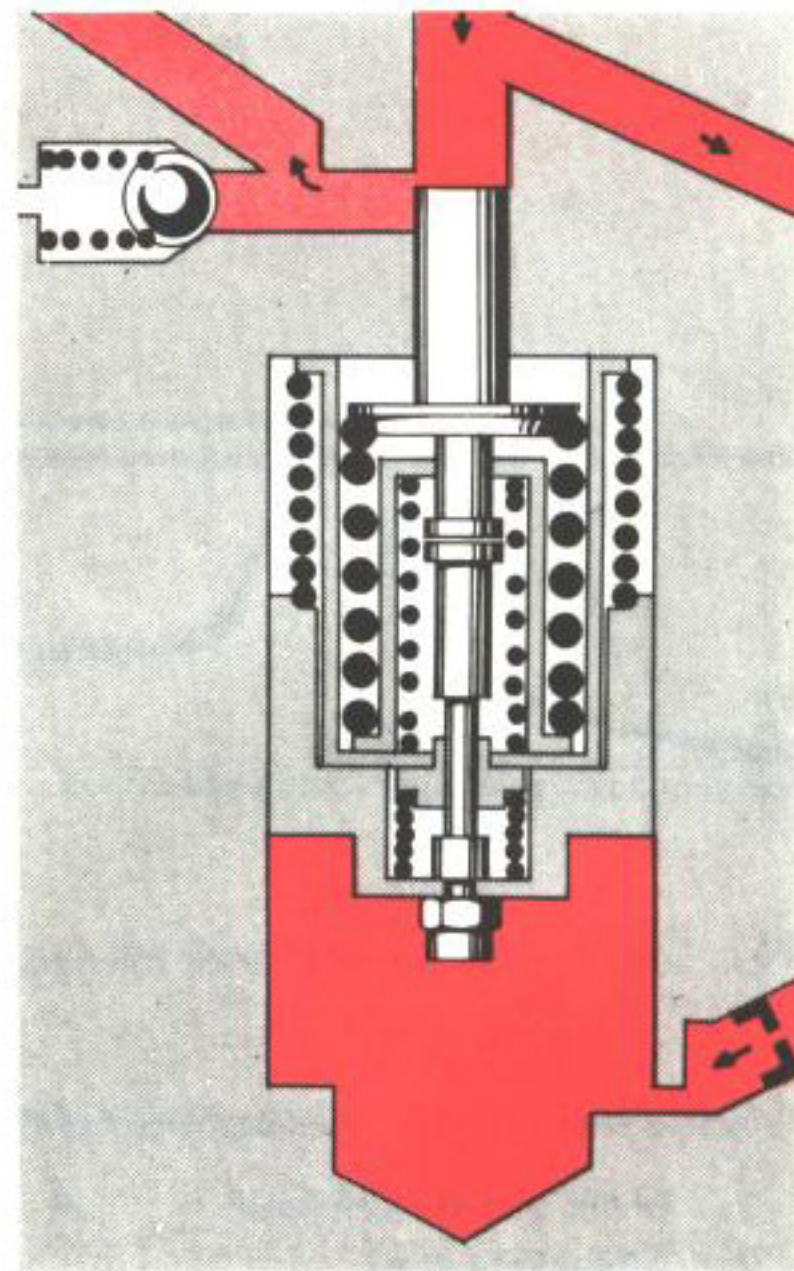
Bild 11. Reducerventil vid överväxel
