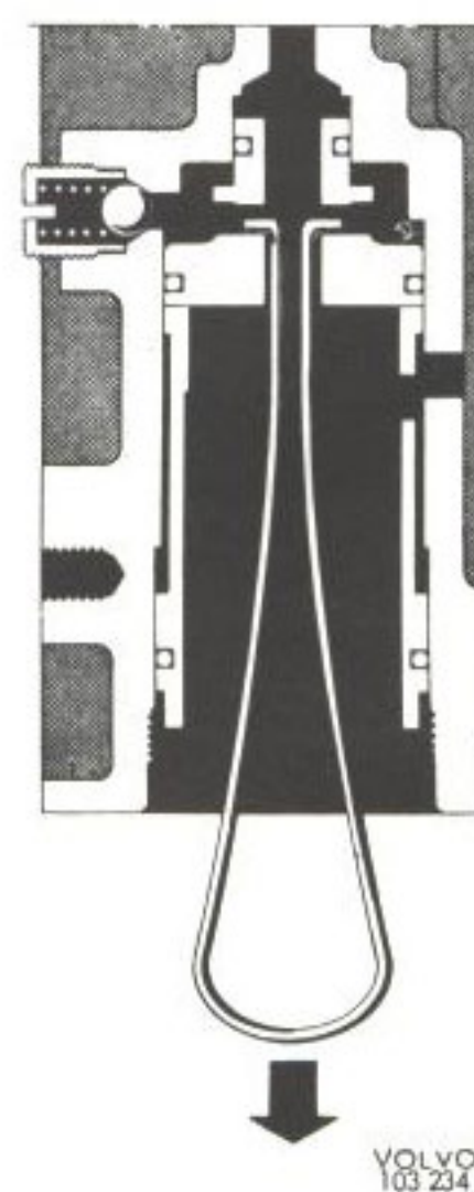
Bild 19. Demontering av reducerventil
