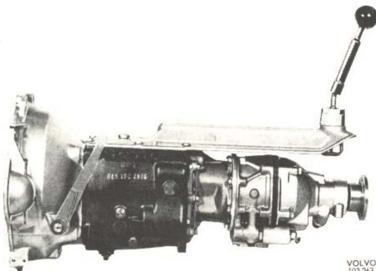
Bild 2. Växellåda M410
