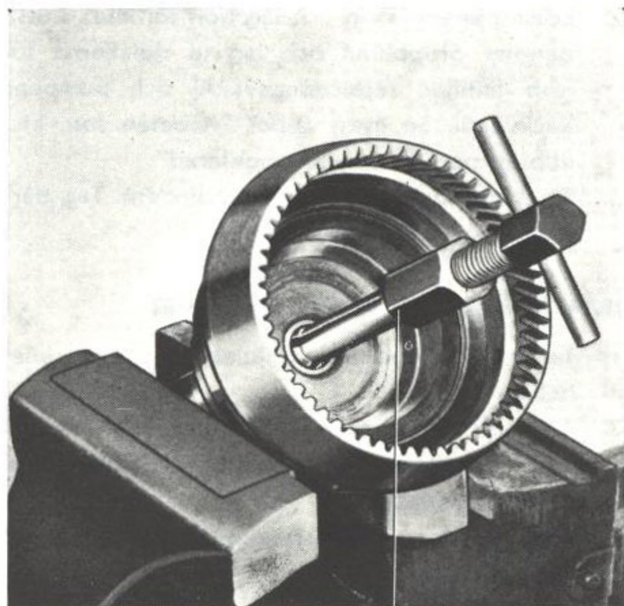
Bild 23. Demontering av bussning, utgående axel
