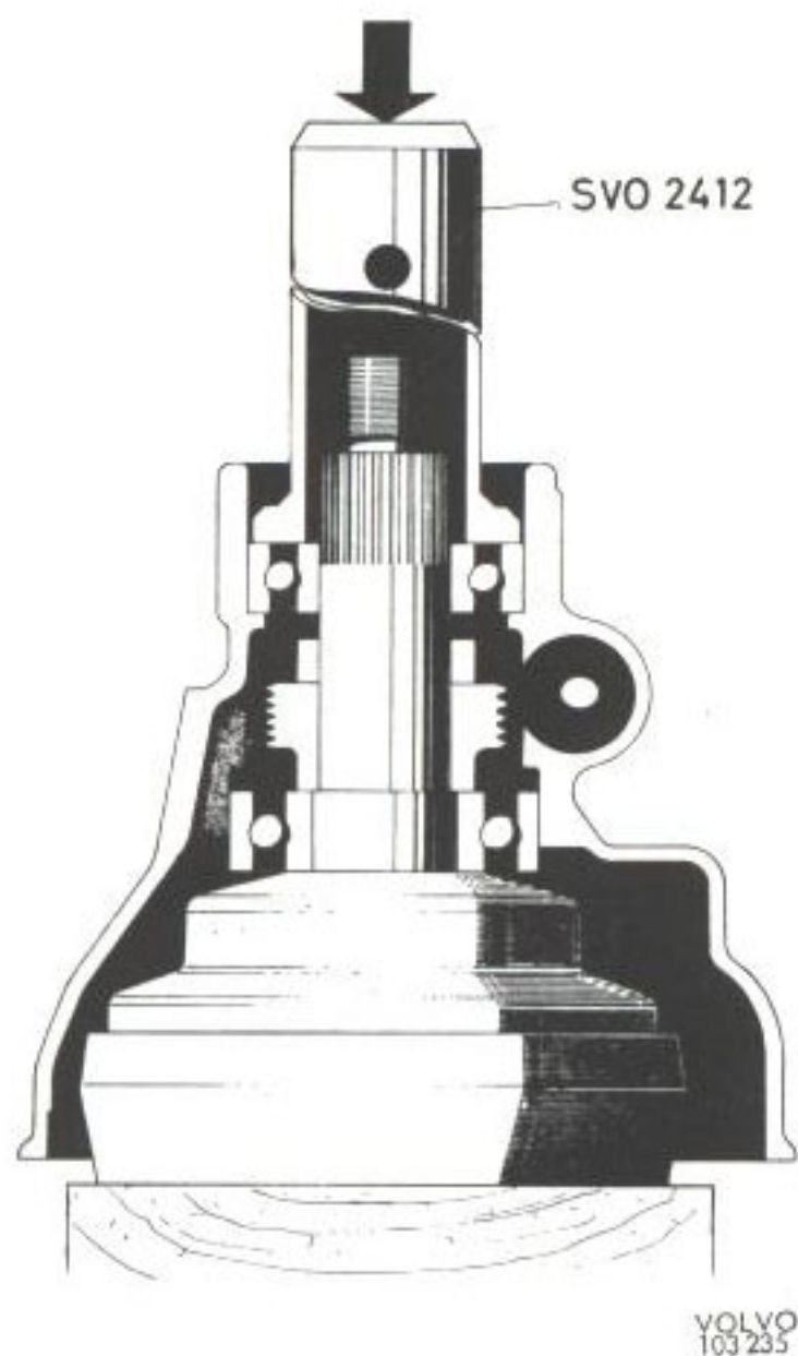
Bild 26. Montering av utgående axel
