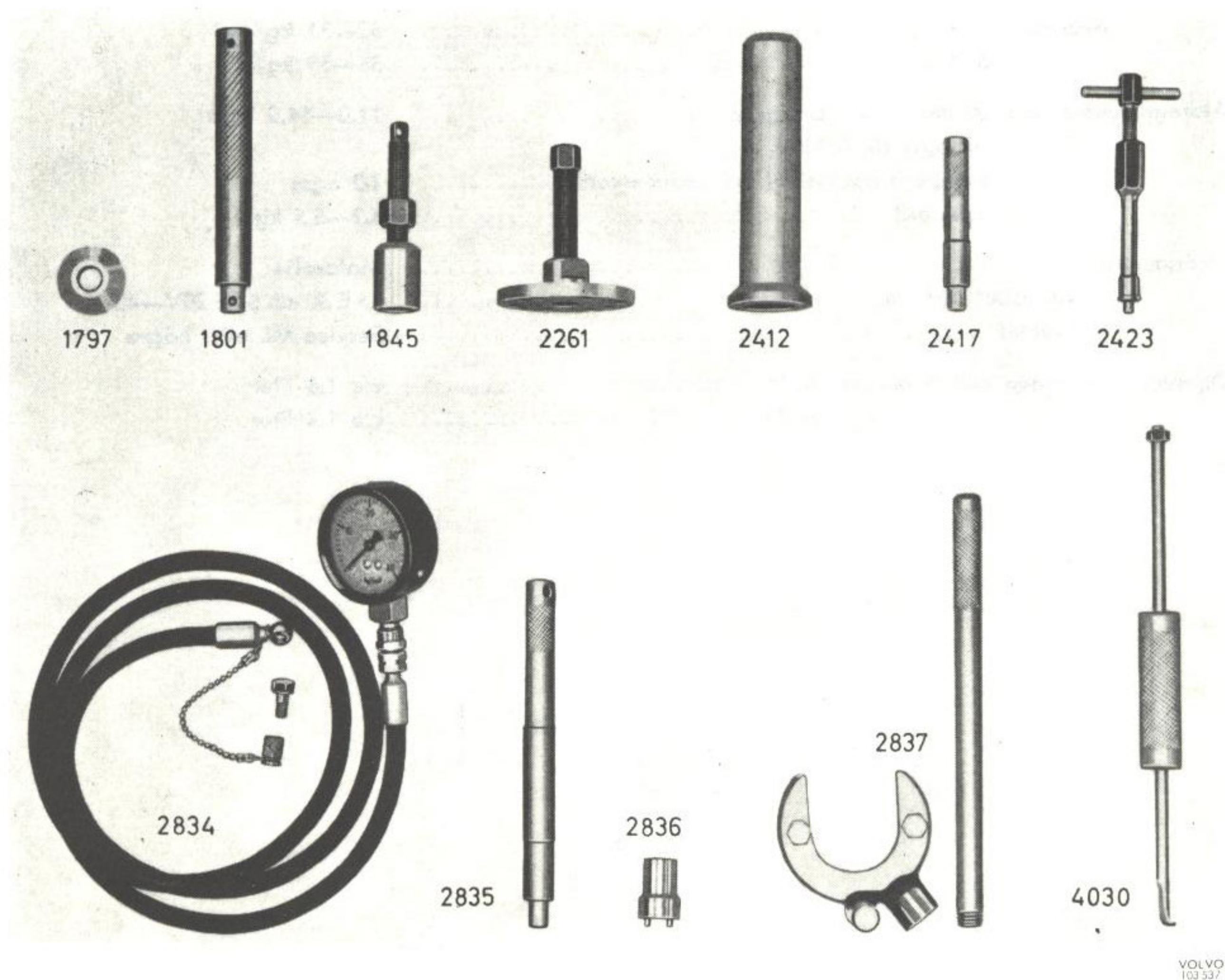
Bild 1. Specialverktyg
