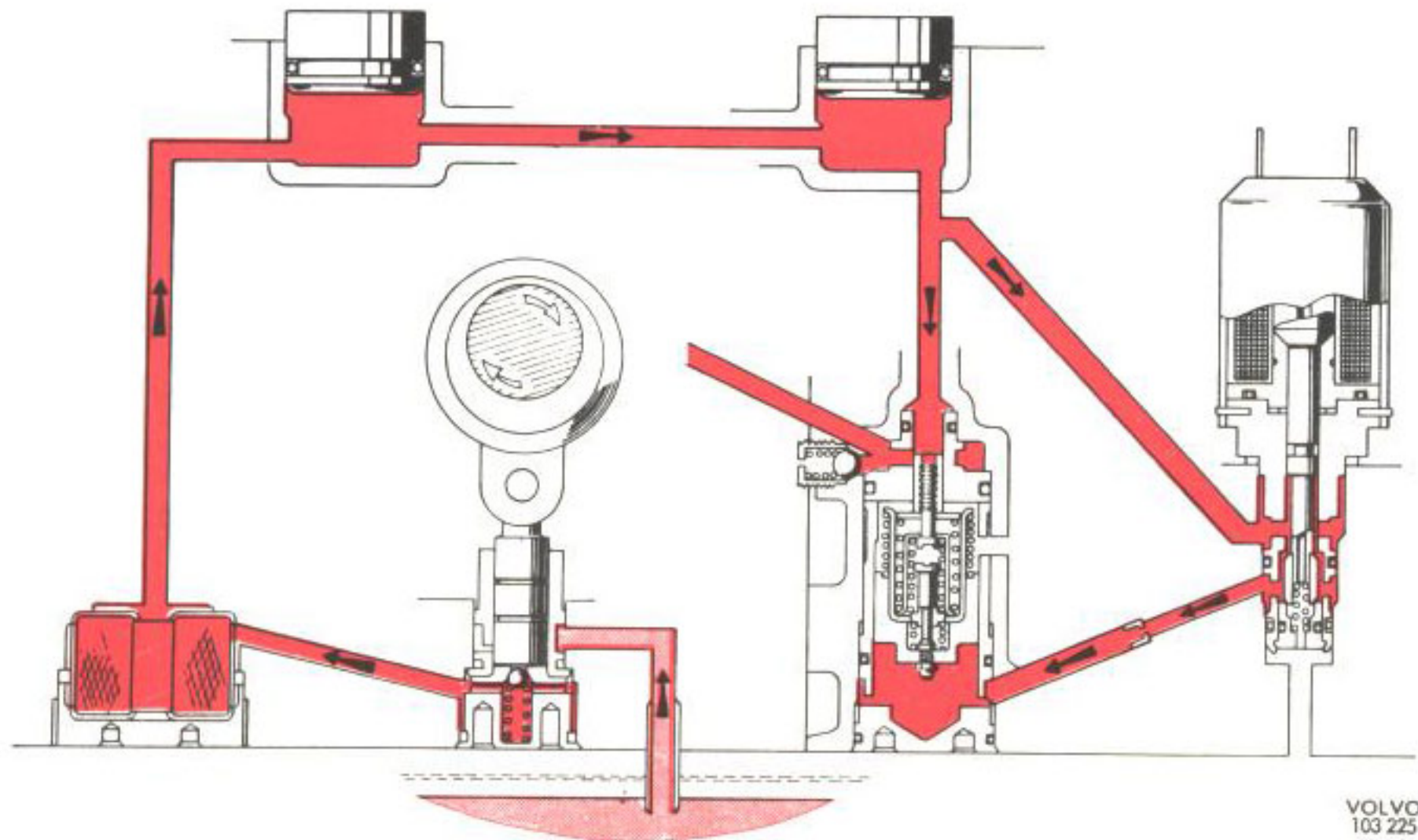
Bild 12. Funktion vid överväxel
