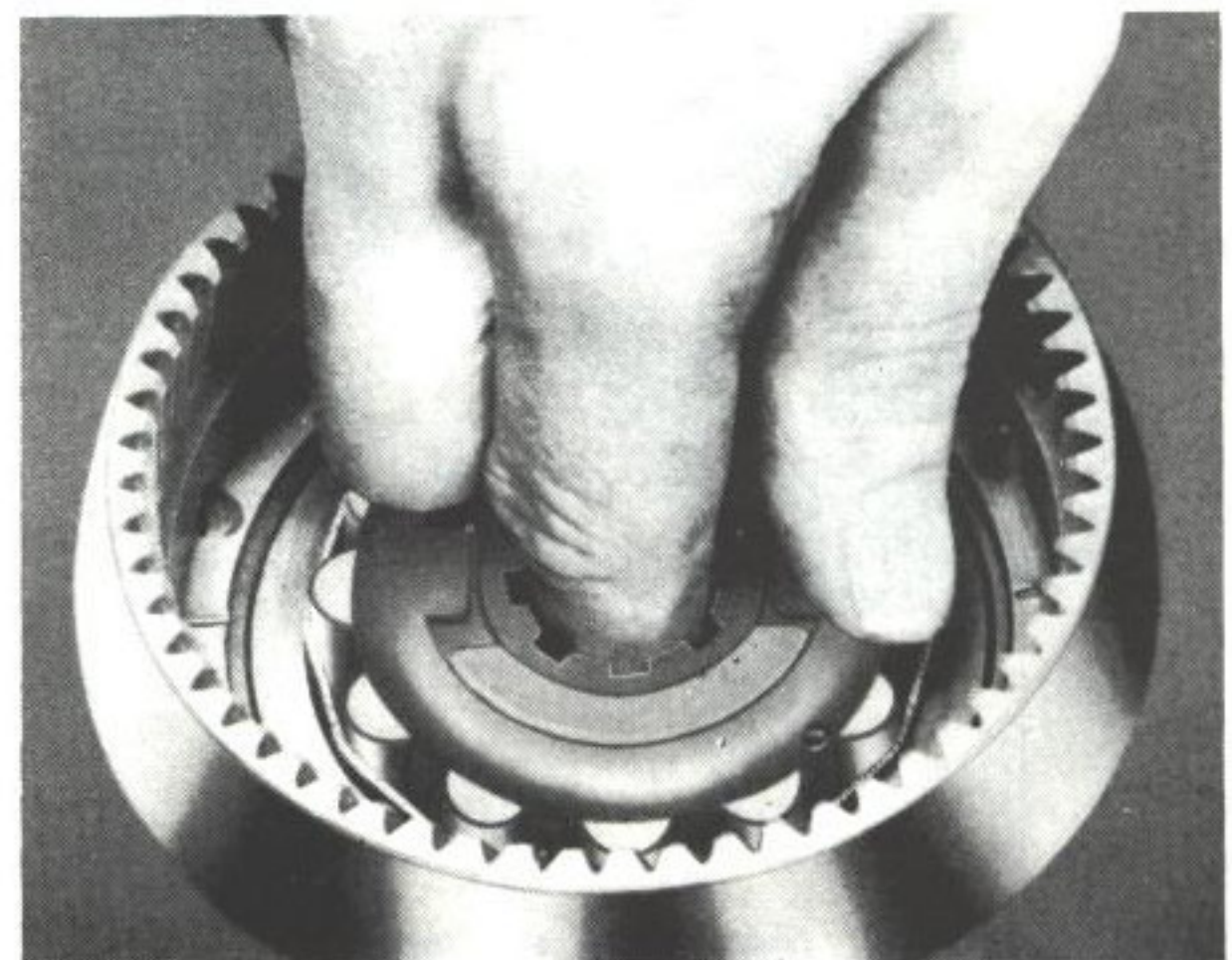
Bild 29. Montering av frihjul
