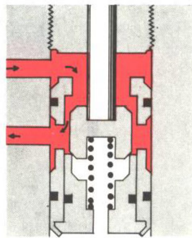
Bild 10. Manöverventil vid överväxel
