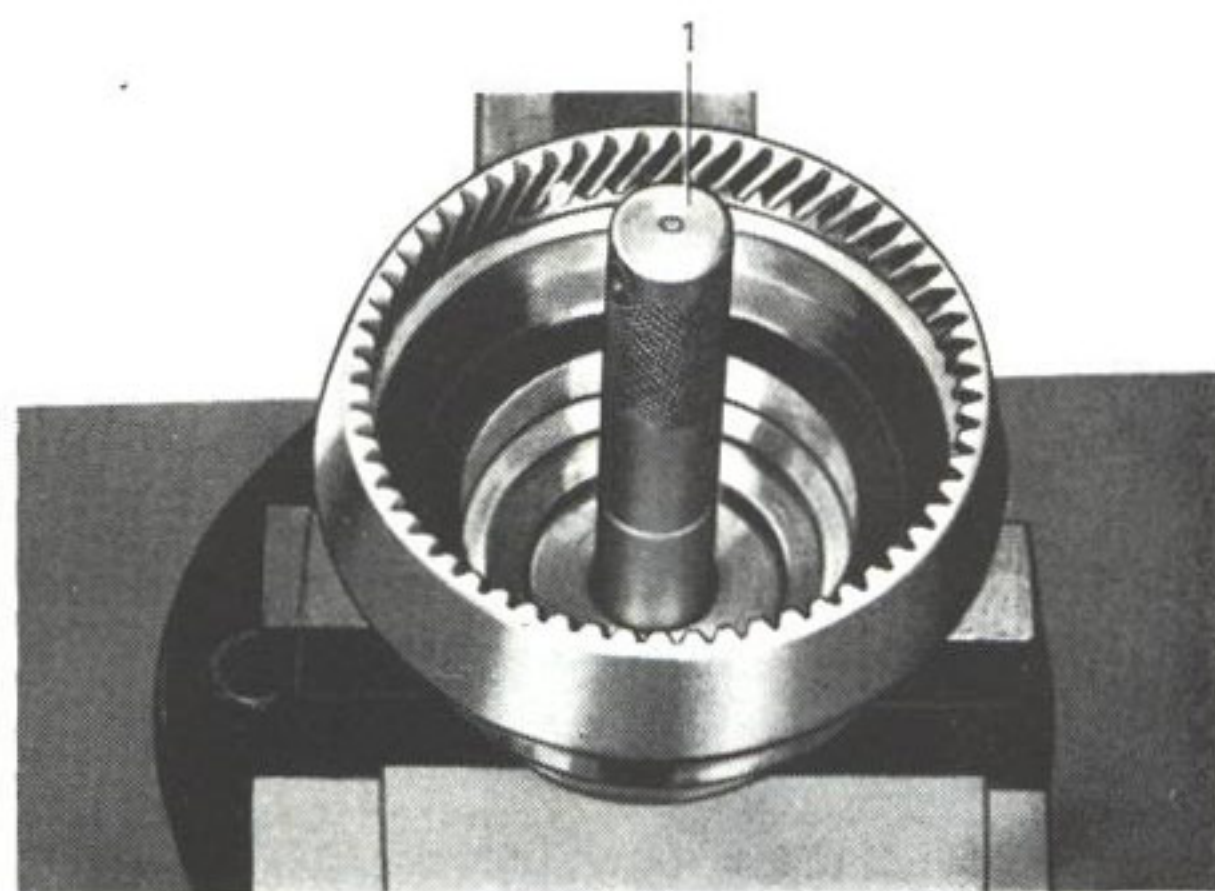
Bild 25. Montering av bussning, utgående axel
